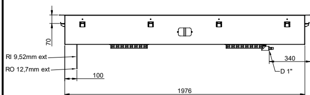
Planta
